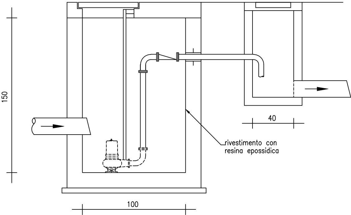
SEZIONE scala 1:20
