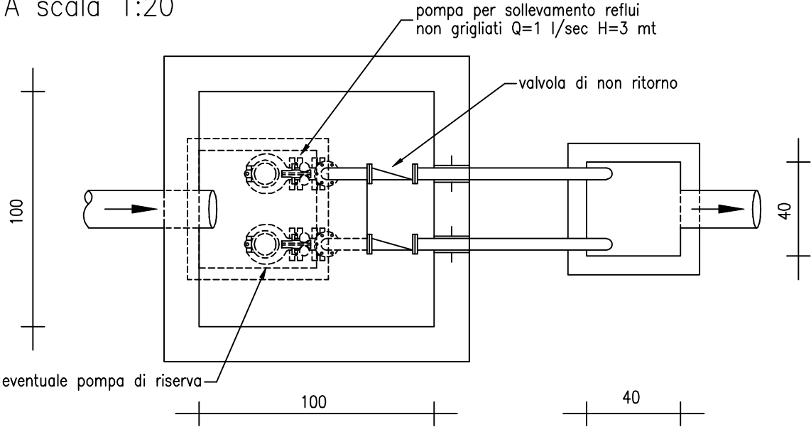
PIANTA scala 1:20
