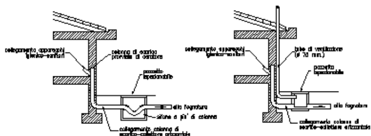
5) fabbrica sprovvista di aeratore su condotta di scarico
