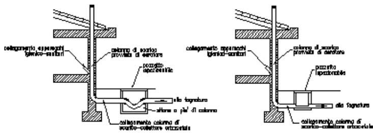
4) fabbrica provvista di aeratore su condotta di scarico
